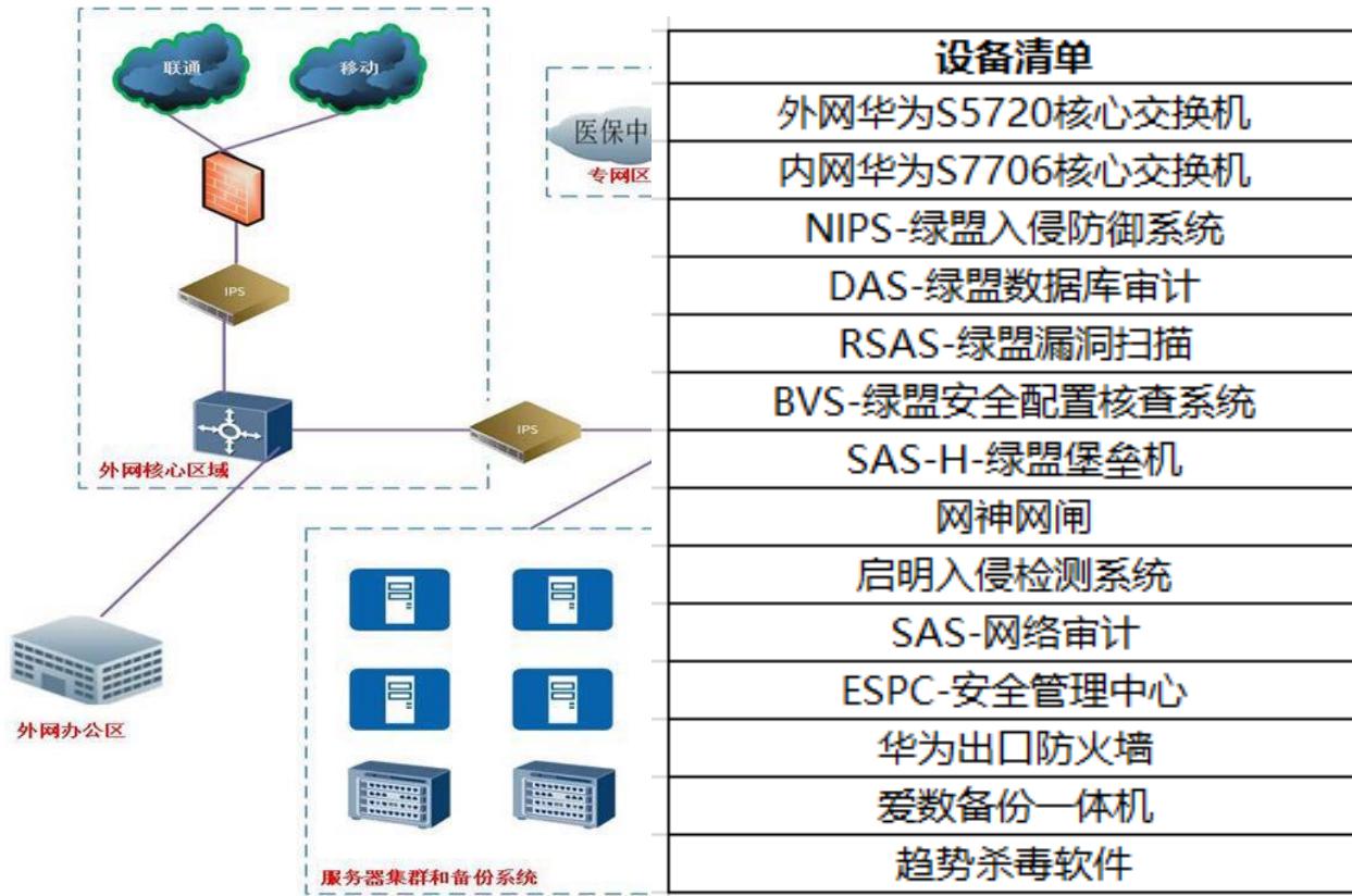
XX医院内网拓扑示意图
